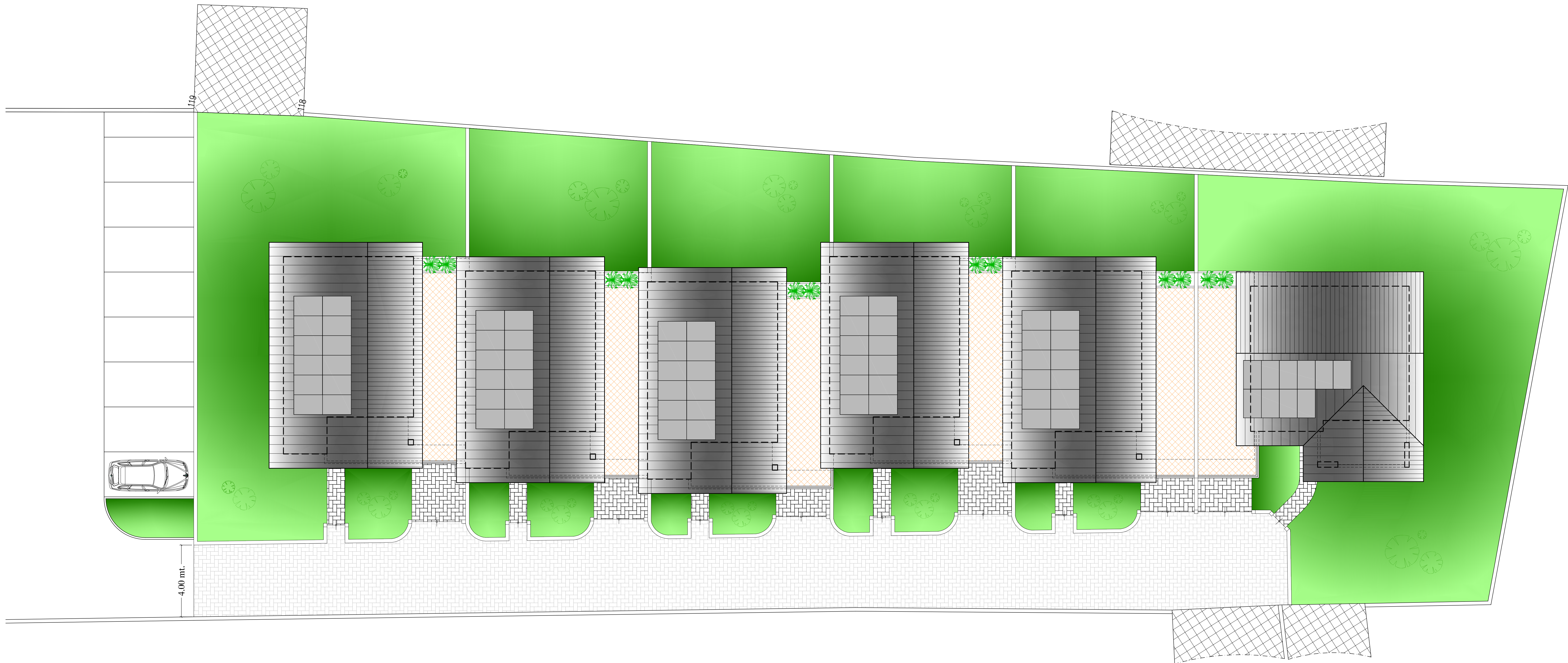
PLANIMETRIA GENERALE 1:100
